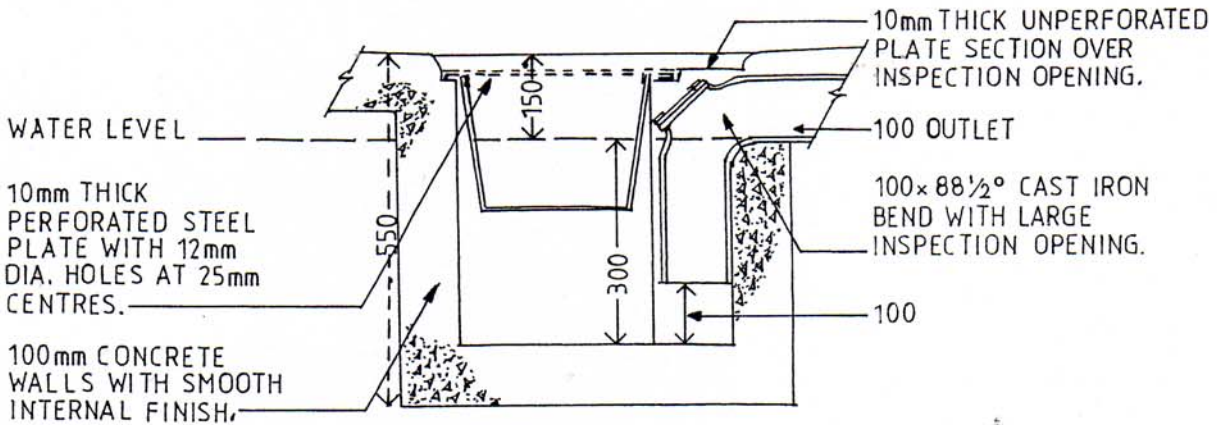
SECTION A-A
